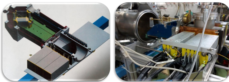
Figura 3.2 – A la izquierda, vista de la cámara actual MAGISOL Si-Plug-in Chamber junto con el soporte y los amplificadores. A la derecha una foto real tomada durante uno de los experimentos siguientes al descrito en esta tesis.
