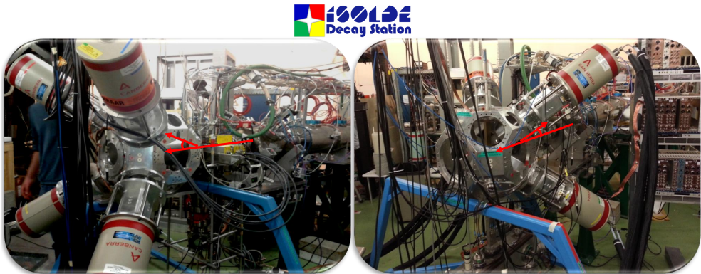
Figura 2.5 – Cambio de configuración de los clovers en la IDS. A la izquierda, su posición en 1977, uno de los primeros experimentos, a ángulos hacia delante con respecto al haz y a la derecha su posición definitiva, a ángulos hacia atrás.
