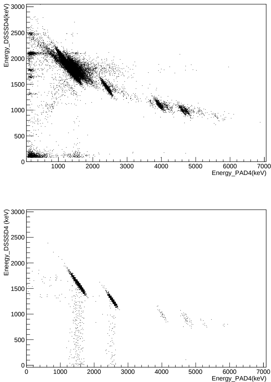
Figura 9.2 – En la parte superior de la figura se muestra el espectro bidimensional en el que se representan las energías de los detectores que forman el telescopio DSSD4 y PAD4 ( 67\ \mu\text{m} ) del dispositivo experimental. En la parte inferior de la figura se muestra el mismo espectro bidimensional que resulta de la simulación con GEANT4. Nótese que solo hemos introducido en la simulación los protones más intensos de la desintegración de ^{33}\text{Ar} . Vemos como el espectro simulado reproduce los datos experimentales.
