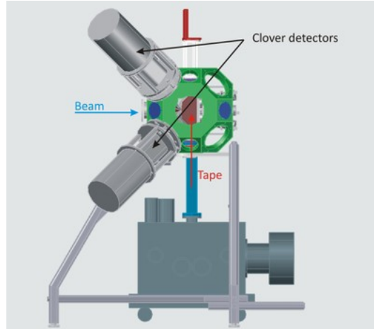
Figura 2.4 – Componentes de la IDS: el soporte de apoyo de toda la estructura (color gris) y el soporte poliédrico para los clovers (verde) de IFIN-HH Bucharest, la tape Station de K.U. Leuven y los propios clovers, dos de ellos de IFIN-HH y los otros dos de K.U. Leuven. Foto tomada de [Leu12]
