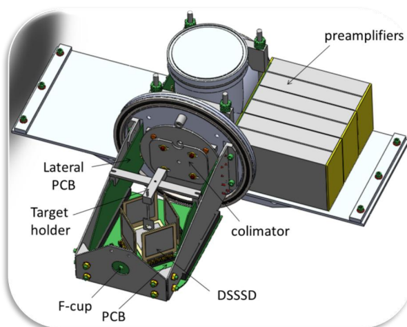
Figura 2.6 – Imagen en 3D de la cámara de detección MAGISOL Si-Plugin Chamber . Cortesía de A.Perea
