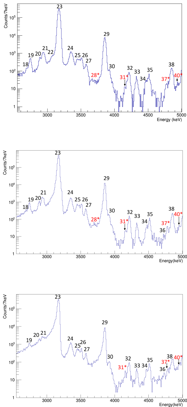
Figura 6.6 – Espectros de los detectores gruesos con la identificación de las transiciones de protones en el intervalo de media energía. De la parte superior a la inferior de la figura, se muestran los espectros de DSSD1 (295 \mu\text{m} ), DSSD2 (524 \mu\text{m} ) y DSSD5 (1000 \mu\text{m} ) respectivamente.
