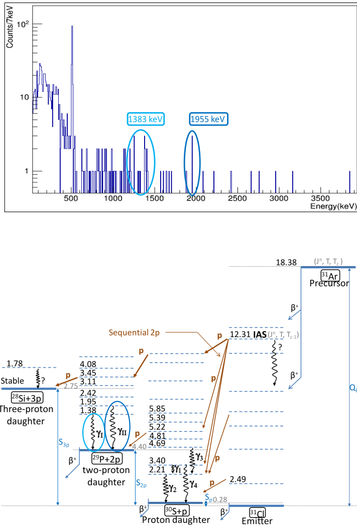
Figura 7.18 – En la parte superior, espectro gamma resultante de la coincidencia de 2 protones con cualquier gamma. Las transiciones gamma de 1383(4) keV y 1954(4) keV han sido identificadas en el esquema de niveles de la desintegración de ^{31}\text{Ar} , mostrado en la parte inferior de la figura.
