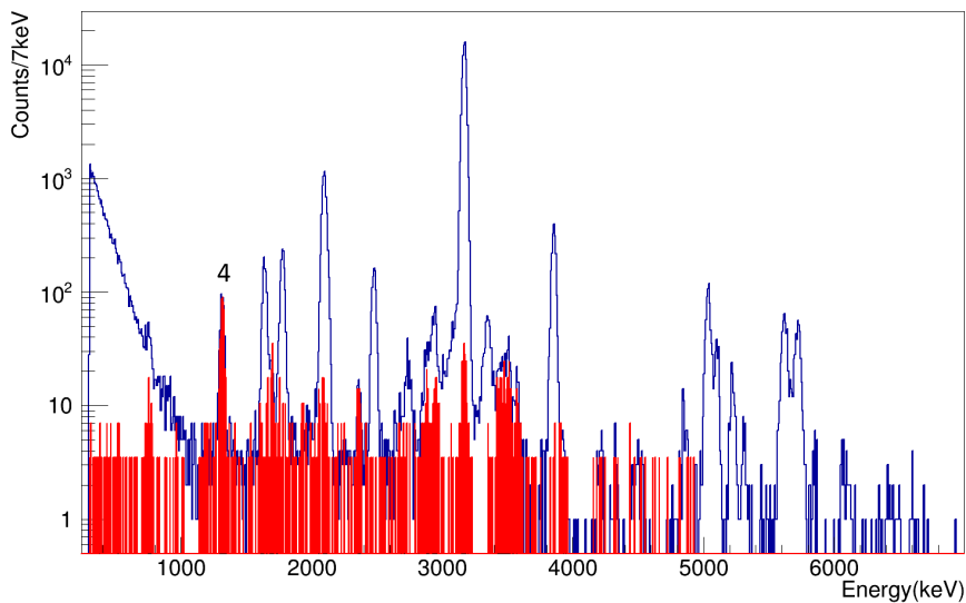
Figura 6.16 – Espectro resultante de las coincidencias beta-protón (color azul) de DSSD1+PAD1, junto con el espectro de coincidencias protón-gamma (color rojo) en el que están incluidos todos los detectores (el mismo del apartado anterior). Este último ha sido escalado usando la transición de protones a 1319 keV con un factor de 3.5. Se observa que el espectro de coincidencias de gamma-protón está dominado por dicha transición.
