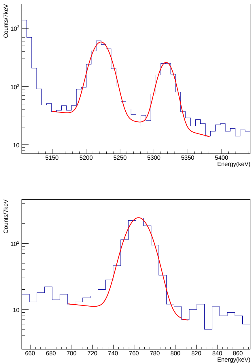
Figura 6.21 – Diferentes ajustes gaussianos con fondo lineal de distintas transiciones en la desintegración de ^{33}\text{Ar} . En la parte superior de a figura, ajuste doble gaussiano de dos transiciones a 5223 keV y 5318 keV del espectro del detector DSSD2. En la parte inferior, ajuste gaussiano de la transición a 765 keV del espectro del detector DSSD4.
