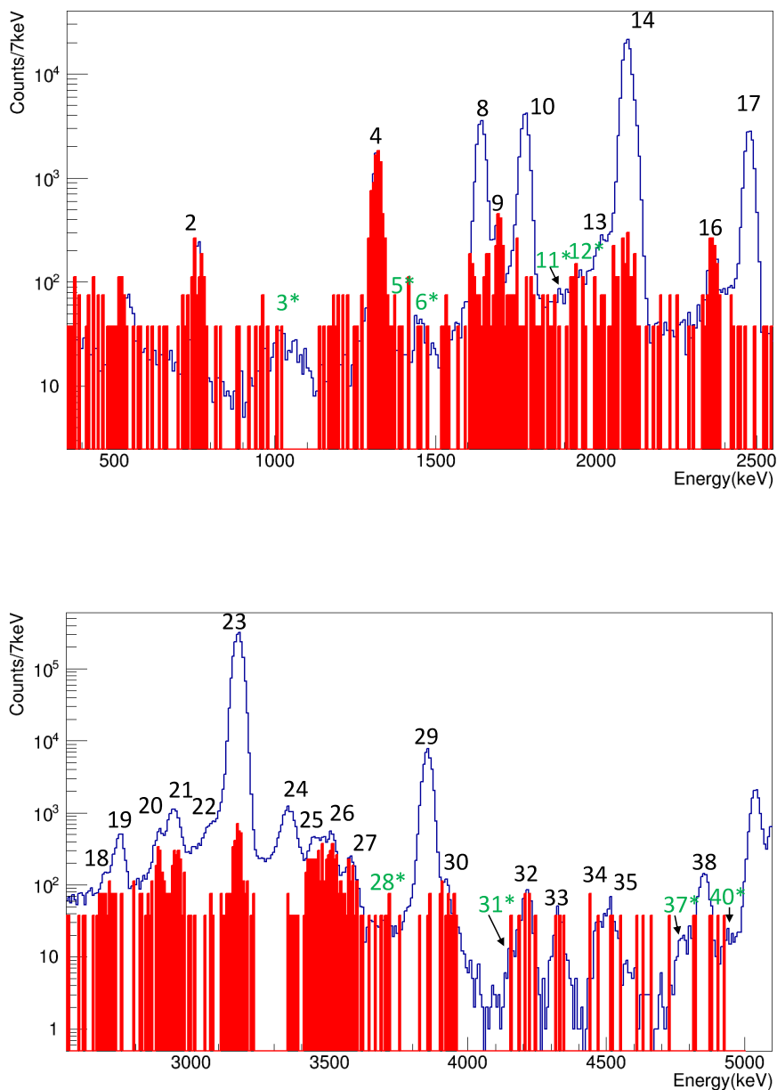
Figura 6.12 – En la parte superior de la figura se muestra el espectro de protones del telescopio DSSD4+PAD4 (color azul) y el espectro de protones que resulta de la coincidencia de todos los detectores de Si con todos los detectores de Ge con una ventana energética centrada en la transición gamma de 2229 keV (color rojo). El espectro de coincidencias ha sido escalado de forma que las áreas del pico correspondiente a la transición de protones de 1317 keV de este y el espectro directo coincidan exactamente. El factor de escala obtenido experimentalmente coincide con el cálculo obtenido por la fórmula 6.3, que en este caso es 34. En la parte inferior de la figura se muestra el espectro de protones y el de coincidencias con la misma gamma de 2229 keV del telescopio DSSD1+PAD1 (color azul). En este caso, el factor de escala es 50. Es mucho más mayor que en el caso anterior, puesto que el ángulo sólido de DSSD1 en este caso es mayor al de DSSD4, en el que solo seleccionamos la región central del detector.
