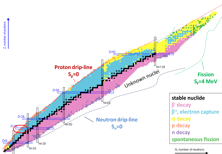
Figura 1.1 – Tabla de nucleidos diagrama de Segré donde se encuentran representados todas las especies nucleares conocidas en función de su número de protones (Z) y neutrones (N). Son identificadas según sus modos de desintegración, que siguen un código específico de colores. Las dos líneas de goteo de protones y neutrones así como la línea donde se anula la barrera de fisión marcan el límite de estabilidad, de forma que el espacio en blanco entre éstas y la zona coloreada, es el ocupado por los nucleidos predichos todavía no conocidos. El círculo rojo marca la situación de los núcleos de interés de este trabajo. Tabla tomada de [NNDC14]
