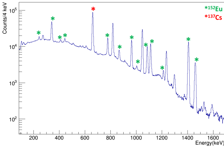
Figura 5.9 – Espectro gamma con las fuentes de calibración ^{152}\text{Eu} y ^{137}\text{Cs} . En la medida de calibración se colocaron las dos fuentes a la vez y en el mismo lugar donde estaba la lámina de implantación durante el experimento. Los asteriscos verdes indican los picos más intensos de la fuente ^{152}\text{Eu} y el asterisco rojo indica el pico más intenso de la fuente ^{137}\text{Cs} .
