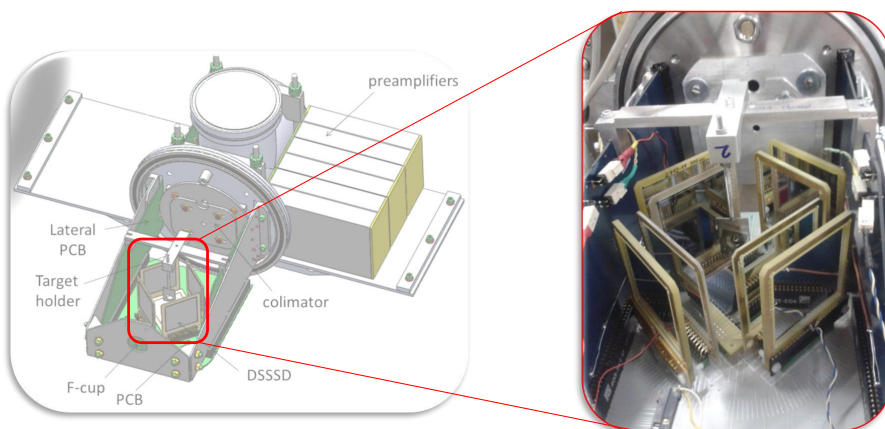
Figura 2.13 – Conjunto de detectores de silicio para partículas cargadas
