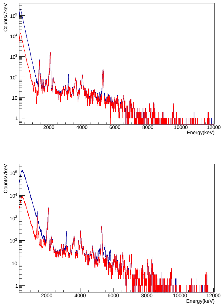
Figura 7.1 – En la parte superior de la figura se muestra los espectros del telescopio DSSD1+PAD1 ( 295\ \mu\text{m} + 1483\ \mu\text{m} ) con la condición en la ventana de tiempo 5-100 ms (espectro color rojo) y sin ella (espectro color azul). En la parte inferior de la figura se muestran los espectros del telescopio DSSD2+PAD2 ( 524\ \mu\text{m} + 1473\ \mu\text{m} ) con las mismas condiciones. Con la condición en la ventana de tiempo, limpiamos el espectro apareciendo los picos 1130 y 1211 keV (color rojo), antes indistinguibles por el fondo beta en el espectro de color azul. Existía contaminación interna de emisores alfa en los detectores de Si, por lo que al poner la condición en la señal de tiempo T1, los picos a 3.18 MeV ( ^{148}\text{Gd} ), 5.1 MeV, 5.45 MeV, 5.85 MeV ( ^{239}\text{Pu} - ^{241}\text{Am} - ^{244}\text{Cm} ) no aparecen en el espectro con la condición en la ventana de tiempo, color rojo.
