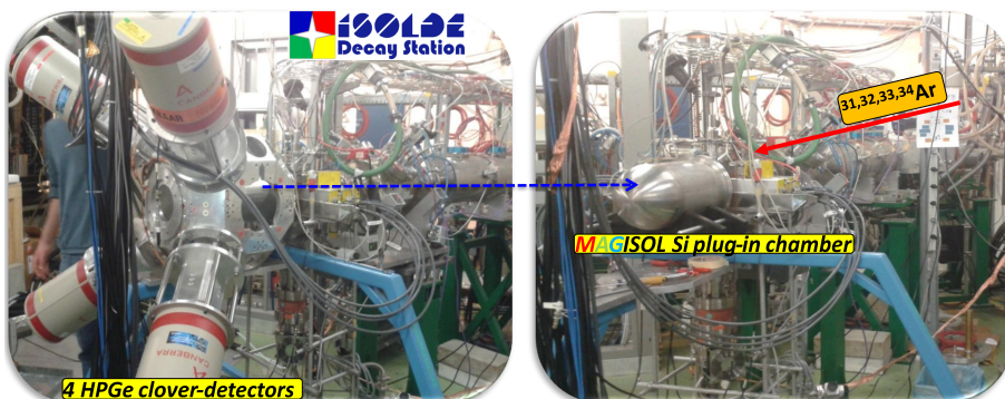
Figura 2.14 – MAGISOL Si-Plugin Chamber en la IDS durante el experimento IS577, donde se muestra el set-up completo, con los clovers de germanio
