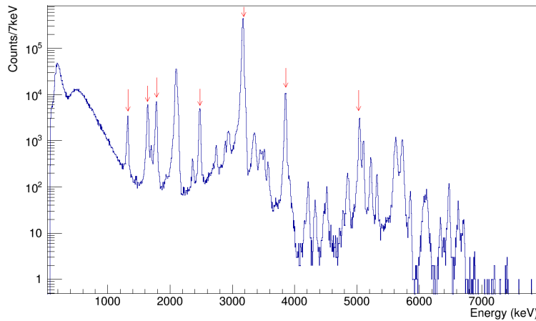
Figura 5.7 – Espectro calibrado de ^{33}\text{Ar} con todas las condiciones anteriores aplicadas correspondiente al DSSD2 (U2, 524 \mu\text{m} ). Las flechas rojas indican todos los picos usados en la calibración de los detectores.
