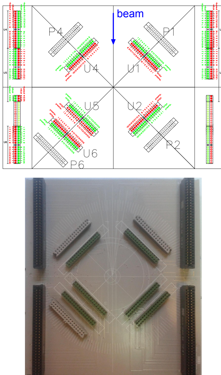
Figura 2.8 – En la parte superior de la figura, se muestra el esquema de la PCB horizontal con las conexiones eléctricas dibujadas. En la parte inferior de la figura, se muestra la PCB horizontal original donde los detectores van conectados.
