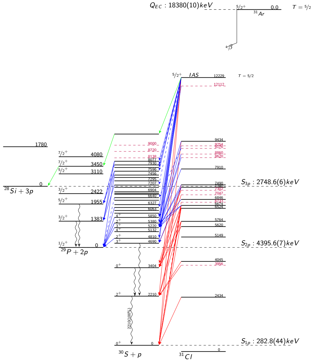
Figura 7.5 – Esquema de desintegración de ^{31}\text{Ar} . En color rojo se muestran las transiciones de protones del canal \beta 1p , en azul se muestra las transiciones del canal \beta 2p y en verde, transiciones implicadas en la emisión de tres protones. Las nuevas transiciones de protones, así como los nuevos estados excitados identificados en este trabajo, se marcan con líneas discontinuas.
