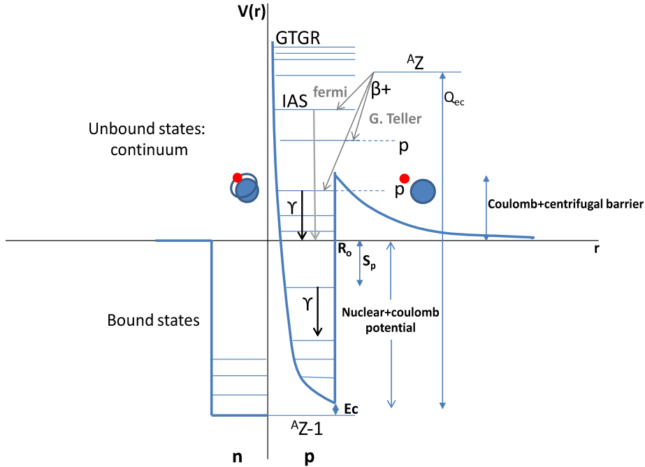
Figura 1.3 – Gráficamente se muestran los estados resonantes que se pueblan tras una desintegración beta en núcleos Z > N . Su desexcitación depende de la barrera coulombiana y centrífuga (si el protón emitido lleva momento angular no nulo). La presencia del potencial coulombiano, hace que el pozo de potencial no sea tan profundo ( E_c , energía de coulomb en el dibujo) como en el caso de los neutrones, eléctricamente neutros. Muy por encima de la barrera solo se da emisión protónica (salvo en el IAS, que también puede desexcitarse por gamma), mientras que en estados justo por encima de la separación hay competición entre gamma y emisión por partículas. Se muestra como la resonancia gigante, análoga al IAS para transiciones Gamow Teller, queda fuera del alcance de la desintegración beta.
