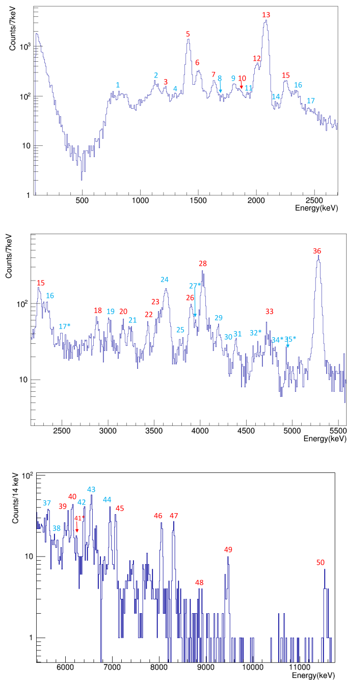
Figura 7.3 – En la parte superior, espectro de protones de DSSD4 (64 \mu\text{m} ) con la identificación de las transiciones de protones a baja energía. En la parte central e inferior, se muestra el espectro de protones del detector DSSD2 (524 \mu\text{m} ) a medias y altas energías, respectivamente. El color rojo indica canal de emisión de un protón y el color azul indica canal de emisión de dos protones. Los asteriscos indican transiciones nuevas identificadas.
