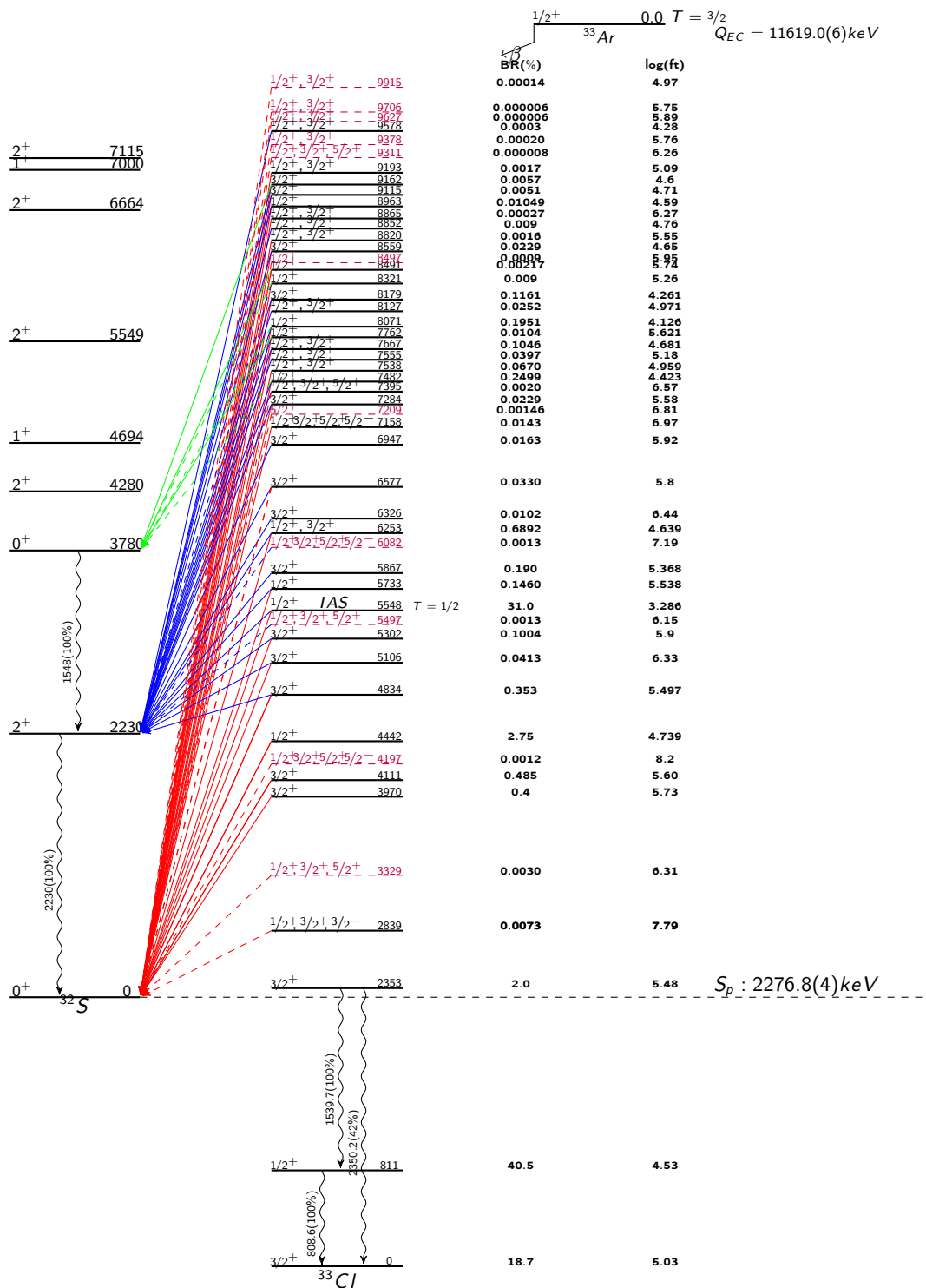
Figura 6.22 – Esquema de desintegración de ^{33}\text{Ar} .
