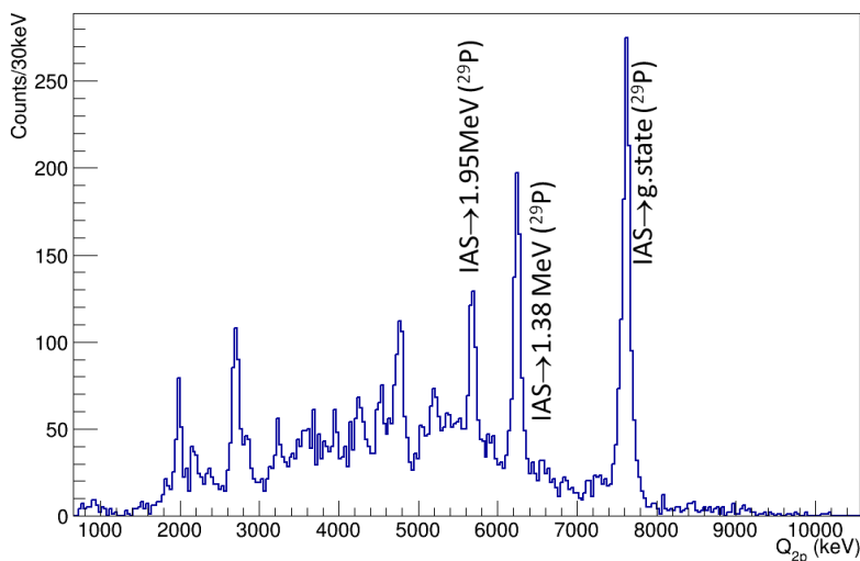
Figura 7.24 – Valores de Q_{2p} para sucesos de emisión de dos protones. Hemos aplicado una energía umbral alta en los detectores para eliminar la contribución beta: E(\text{DSSD1}) > 629 \text{ keV} , E(\text{DSSD2}) > 1020 \text{ keV} , E(\text{DSSD5}) > 2040 \text{ keV} , E(\text{DSSD4}) > 346 \text{ keV} y E(\text{DSSD6}) > 321 \text{ keV} . Las líneas más intensas corresponden a las transiciones desde el IAS de ^{31}\text{Cl} . El resto de líneas corresponden a transiciones desde estados de ^{31}\text{Cl} alimentados por desintegración beta tipo Gamow-Teller, y la mayoría de dichas transiciones tienen como estado final el fundamental de ^{29}\text{P} .
