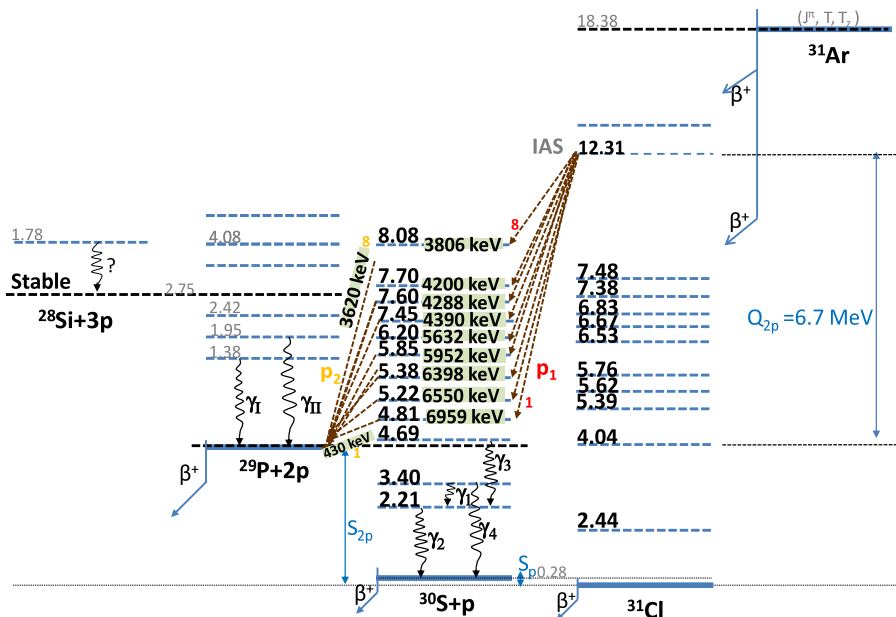
Figura 7.29 – Sucesos de emisión de dos protones de las figuras 7.27 y 7.25 con un valor de Q_{2p} de 6.7 MeV. Se pueblan estados hasta 8 MeV en ^{30}\text{S} .
