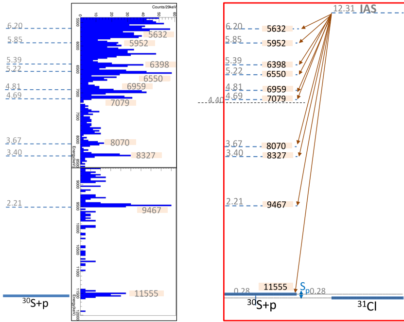
Figura 7.22 – A la izquierda espectro a altas energías del detector horizontal DSSD5 y a la derecha los niveles correspondientes desde los que los protones son emitidos. Vemos que el IAS muestra una gran fragmentación, su desintegración va a numerosos estados finales del núcleo hijo ^{30}\text{S} . Esto hace que los espectros directos de protones presenten una ausencia del pico que domina el espectro y proviene de la desintegración del IAS, a diferencia del caso de ^{33}\text{Ar} .
