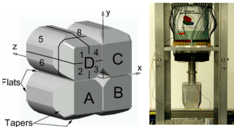
Figura 2.12 – A la izquierda, muestra de un detector de germanio segmentado tipo clover . A,B,C,D indican cuatro cristales de germanio, divididos cada uno en otros cuatro cristales (1-8) por los contactos. A la derecha un detector real, donde se ve el cristal y su criostato de refrigeración con nitrógeno líquido.
